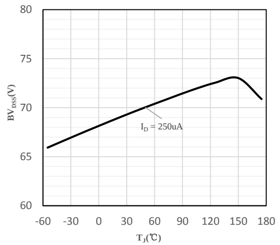
Fig 12 BV_{DSS} vs T_J
